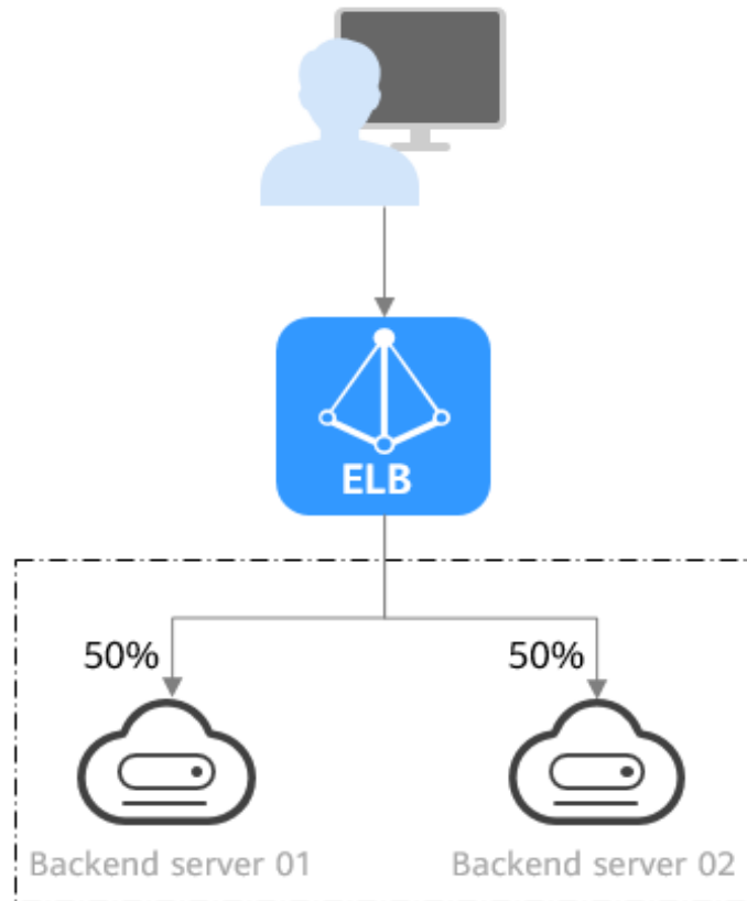
Figura 4-7 Distribución del tráfico utilizando el algoritmo de round robin ponderado
