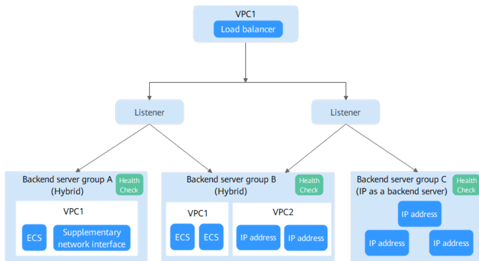
Figura 4-1 Arquitectura de grupo de servidores backend
