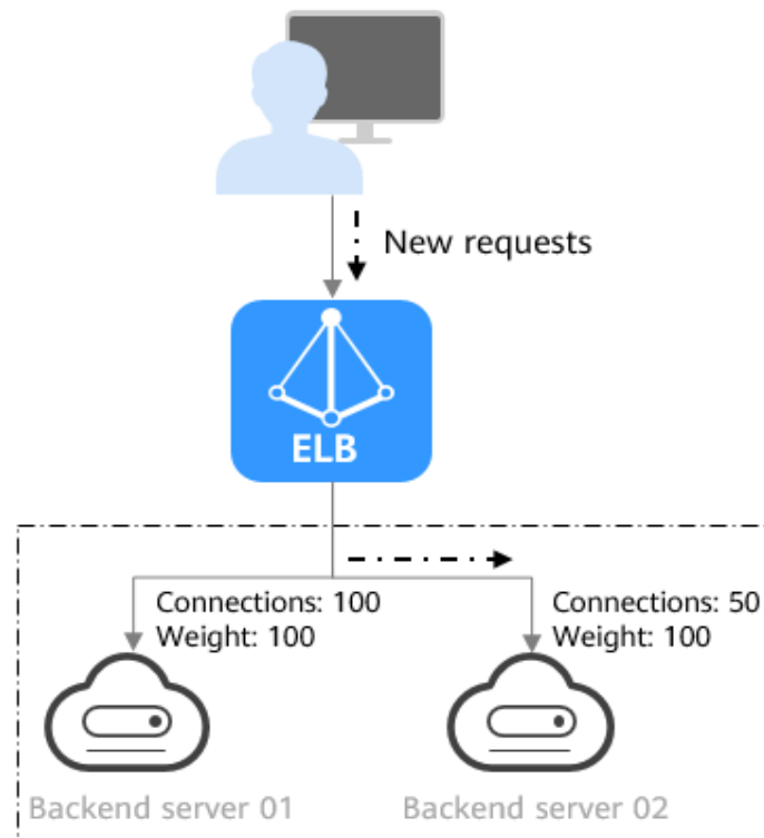
Figura 4-8 Distribución del tráfico utilizando el algoritmo de conexiones mínimas ponderadas
