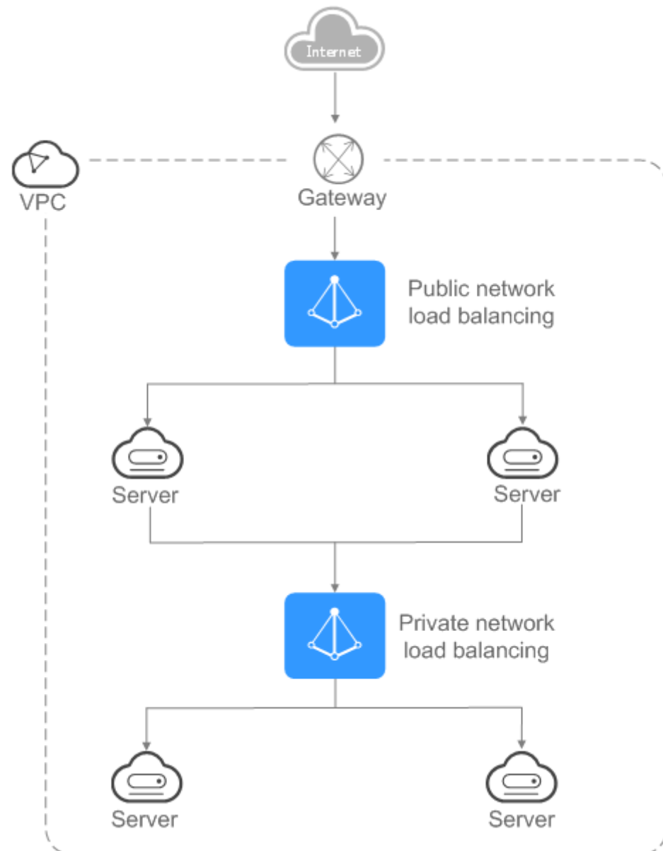
Figura 1-2 Los balanceadores de carga en las redes públicas y las privadas
