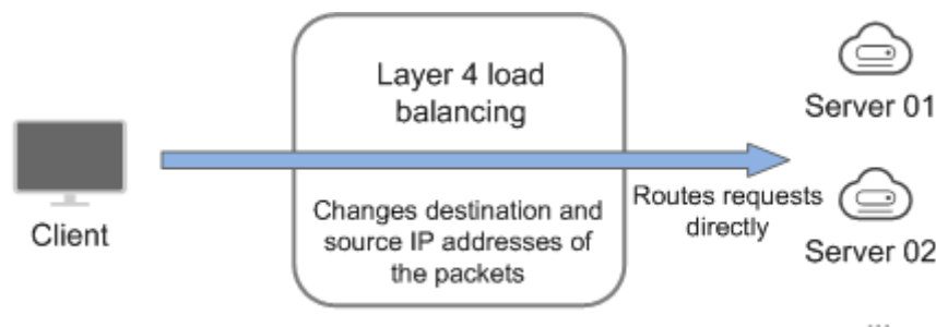
Figura 1-3 Balanceo de carga de capa 4
