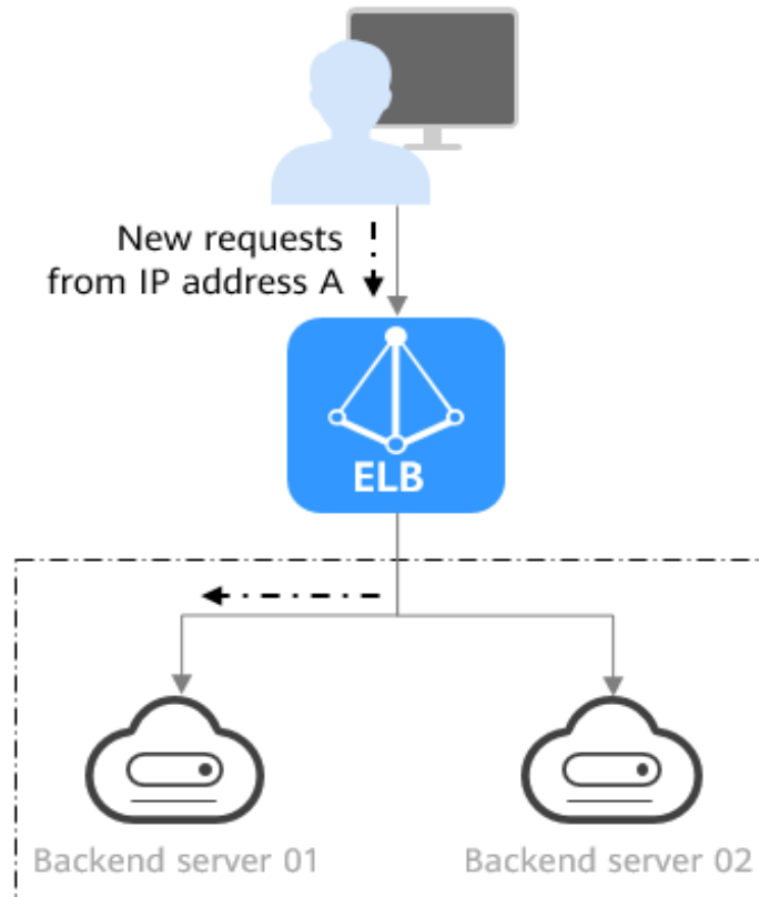
Figura 4-9 Distribución del tráfico mediante el algoritmo de hash IP de origen
