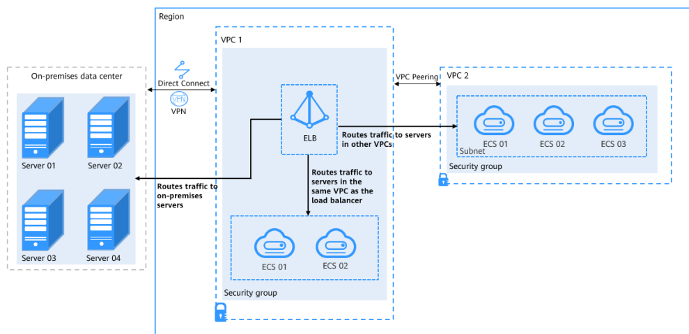
Figura 5-1 Enrutamiento de solicitudes a servidores en la nube y locales
